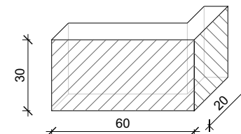
Sarokelem „a” corner element „a” 60x30x20 cm
