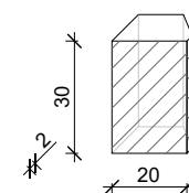
Sarokelem „c” corner element „c” 20x30x10 cm
